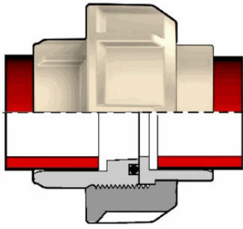
Муфта разборная ПВХ d63 SDR21 PN16
