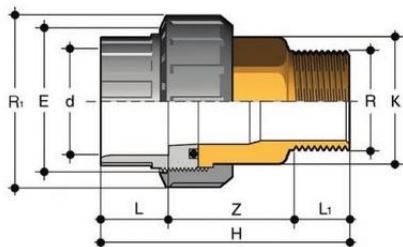
Муфта разборная с НР ПВХ (латунь) FIP 25x3/4
