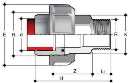
Муфта разборная переходная PP-H / нерж.сталь, HP, (EPDM) FIP 50x1 1/2 PN10
