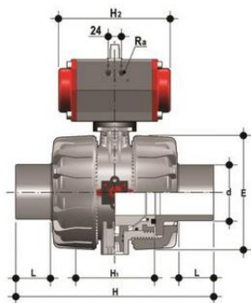
Шаровой кран VKD с пневмоприводом НО с втулочными окончаниями, DN65-100 (уплотнение FKM) PP-H d75 (DN65)
