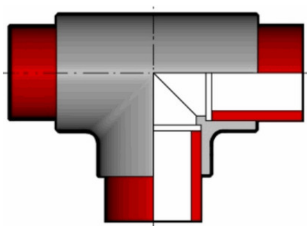
Тройник ПВДФ 90° d25 SDR21 PN16
