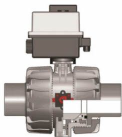
Шаровой кран VKD ПВДФ с эл.приводом 90-240V, втулочные окончания d110 (DN90)
