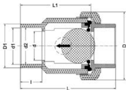
Обратный клапан шаровой с одним разборным соединением, муфтовые окончания PP-H IPS (FKM) d63 (DN50)
