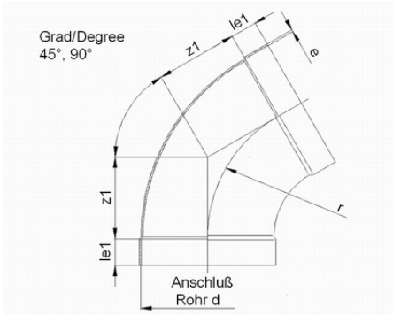
Изгиб 45° PPs d180
