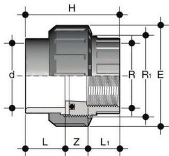
Муфта разборная с ВР ПВХ FIP 32x1
