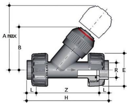
Угловой обратный клапан VRUFV ПВХ с резьбовыми окончаниями, EPDM, FIP R1/2" (DN15)
