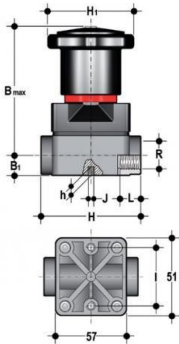
Компактный мембранный клапан CM ПВХДФ с резьбовыми окончаниями R3/8" (DN12)
