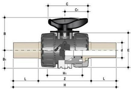
Шаровой кран для регулирования потока VKR с патрубками (CVDM) (уплотнение EPDM) PP-H d63 (DN50)
