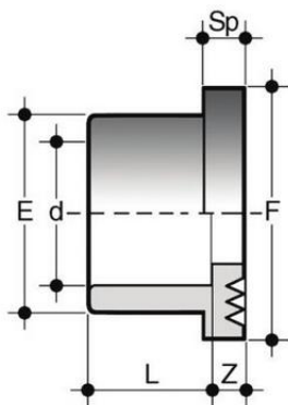
Бурт с зубчатой поверхностью ПВХ FIP d200
