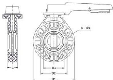
Дисковый затвор IFK ПВДФ с рукояткой d90 (DN80)
