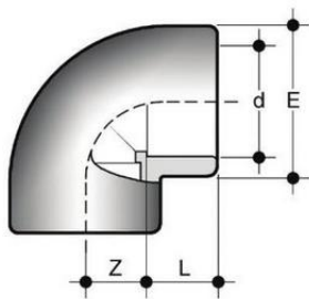
Отвод 90° ХПВХ d110 PN16
