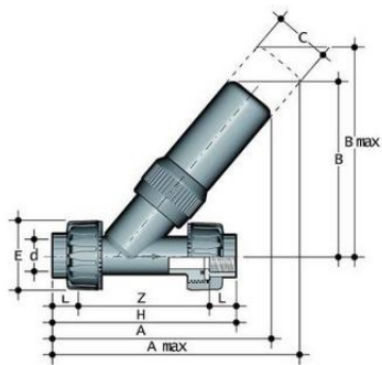
Угловой предохранительный клапан SV PBX с резьбовыми окончаниями, FKM, FIP R1" (DN25)
