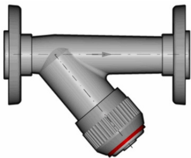
Грязевый фильтр RVOT PBX с фланцевыми окончаниями, EPDM, FIP d32 (DN25)
