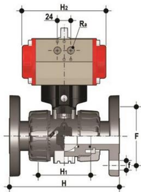
Шаровой кран VKD ХПВХ с пневмоприводом НЗ с фланцевыми окончаниями d40 (DN32)
