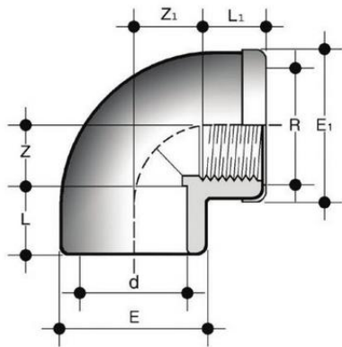
Отвод переходной ВР с усиливающим кольцом ХПВХ 16x3/8" PN16
