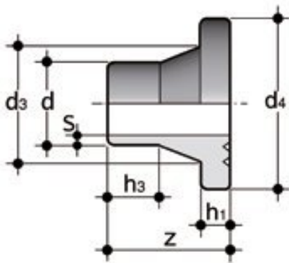
Бурт под фланец для стыковой сварки PP-H FIP (PN6) d110 SDR17.6 PN6
