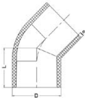
Отвод для стыковой сварки 45° PP-H IPS (Model B) d160 PN10
