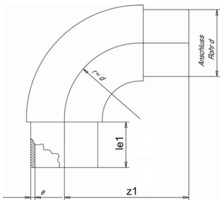
Изгиб 90° PP-H Simona d25 SDR11 PN6
