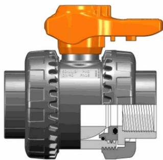
Шаровой кран общего применения VXE ХПВХ с резьбовыми окончаниями R3/4" (DN20)
