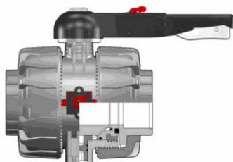
Шаровой кран промышленного применения VKD ХПВХ с муфтовыми окончаниями, DN65-100 d90
