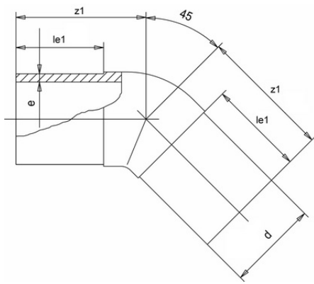
Отвод ПВДФ 45° (Simona) d32 SDR21 PN16
