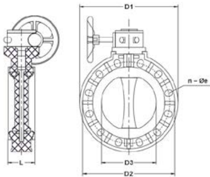
Затвор дисковый промышленный с редуктором ХПВХ IPS (Model B) d40"(DN1000)
