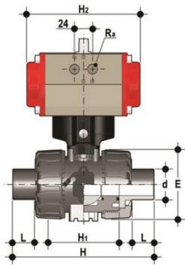
Шаровой кран VKD ХПВХ с пневмоприводом НО с втулочными окончаниями d25 (DN20)
