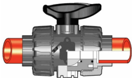
Шаровой кран промышленного применения VKD с муфтовыми окончаниями (уплотнение EPDM) PP-H d25
