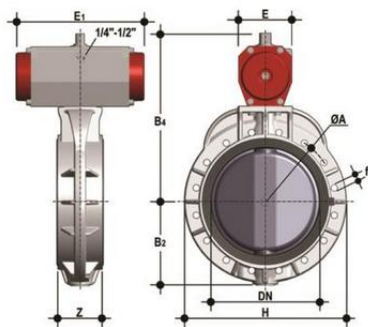
Дисковый затвор FK с пневмоприводом НО (уплотнение FKM) PP-H d355 (DN350)
