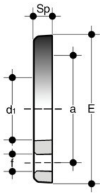
Свободный фланец ПВХ FIP d140
