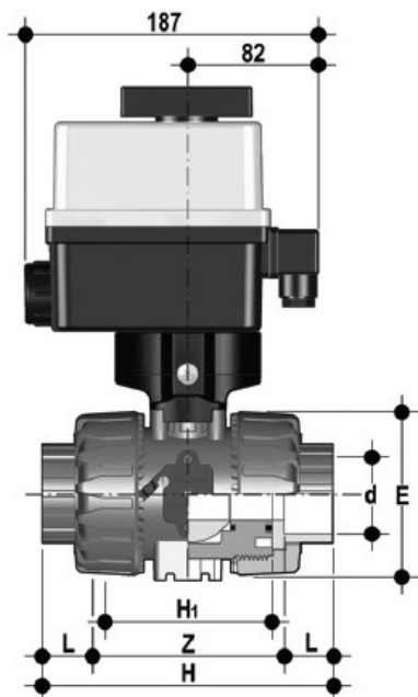
Шаровой кран VKD ПВХ с эл.приводом 90-240V, муфтовые окончания, EPDM, FIP d16 (DN10)
