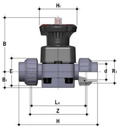
Мембранный клапан ДК ПВХ с муфтовыми окончаниями d63 (DN50)
