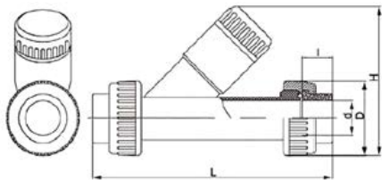
Фильтр сетчатый ХПВХ IPS d32
