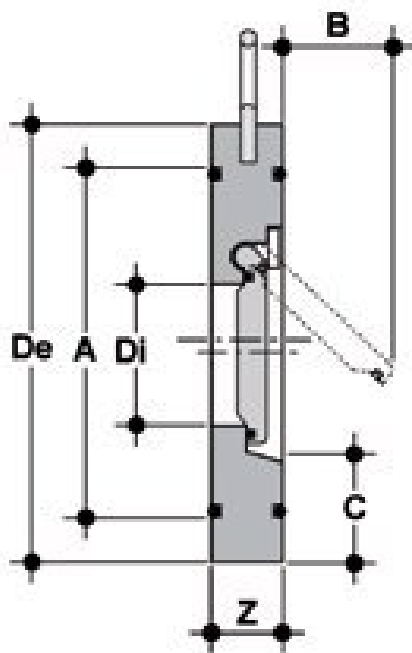
Межфланцевый обратный CROV ПВХ, EPDM, FIP d110 (DN100)
