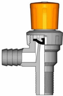
Мембранный кран RMRPV ПВХ, EPDM, FIP d15 (DN15)
