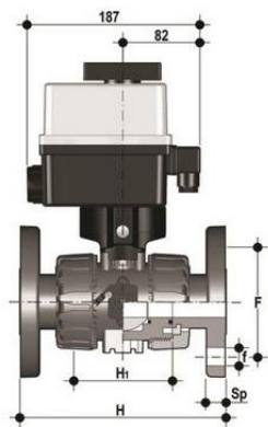
Шаровой кран VKD ПВДФ с эл.приводом 24V AC/DC, фланцевые окончания d50 (DN40)
