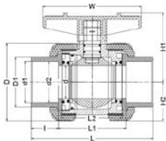
Кран шаровой промышленного применения, муфтовые окончания, EPDM, IPS d90
