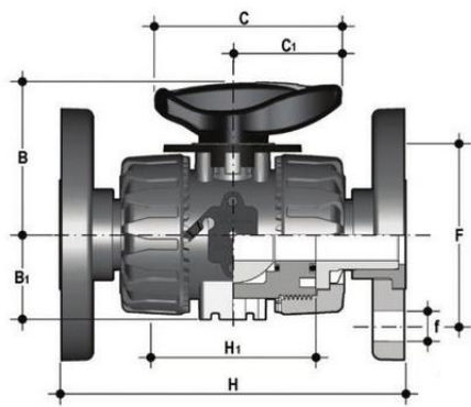
Шаровой кран для регулирования потока VKR с фланцевыми окончаниями (уплотнение EPDM) PP-H d50 (DN40)
