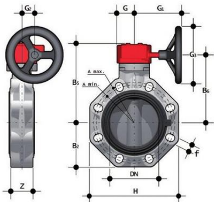
Дисковый затвор FK ХПВХ с редуктором d75 (DN65)
