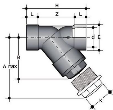
Грязевый фильтр RVIV ПВХ с муфтовыми окончаниями, EPDM, FIP d90 (DN80)
