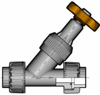
Угловой вентиль VVUIV ПВХ с разборными муфтовыми окончаниями, EPDM, FIP d16 (DN10)
