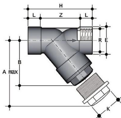
Грязевый фильтр из серого ПВХ с резьбовыми окончаниями, EPDM, FIP R4" (DN100)
