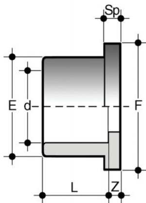
Бурт под фланец ПВХ FIP d75
