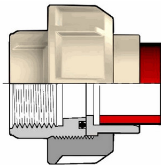
Разборная муфта с ВР, раструбная сварка РР-Н (EPDM) FIP 20x1/2 PN10
