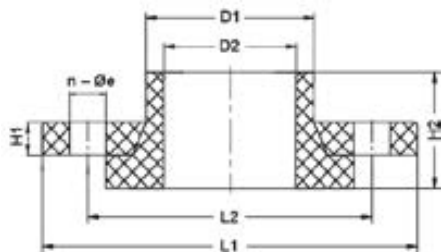
Бурт+фланец (комплект) для стыковой сварки ПВДФ IPS d40 PN 16
