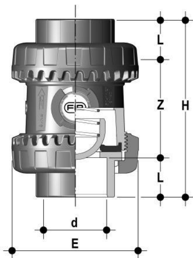
Пружинный шаровой обратный клапан SSEIV ПВХ; с муфтовыми окончаниями, EPDM, FIP d25 (DN20)
