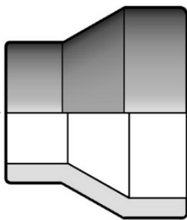
Муфта редукционная для стыковой сварки PP-H FIP 110x63 SDR11 PN6
