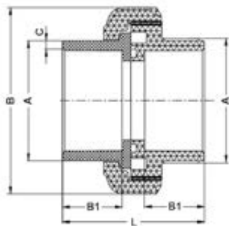
Муфта разборная для стыковой сварки PP-H IPS d25 PN 10
