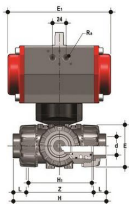
3-х ходовой шаровой кран ТКД ПБХ с пневмоприводом, L-шар, FIP d63 (DN50)
