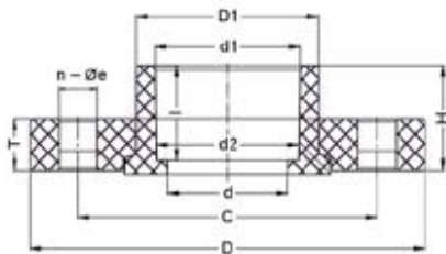
Фланец свободный с буртом ХПВХ IPS (Model A) d32 PN16
